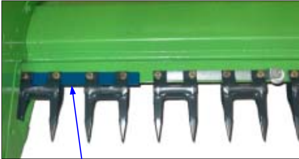
Führungsplatte 4-Loch.
